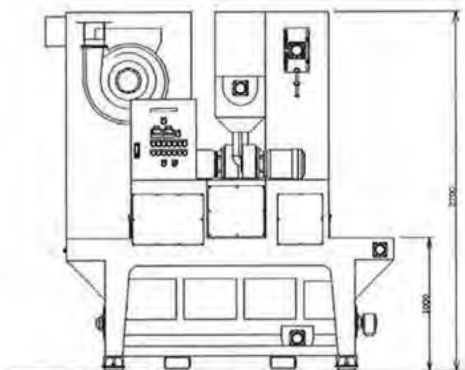
○立面図
